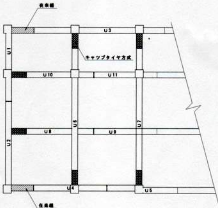
梁ユニット割付図 S=1:100
